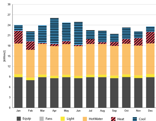
A. Intensidad del uso de energía del caso base
