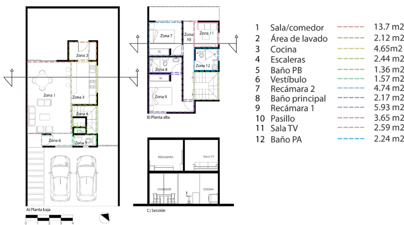
FIGURA 2. ZONAS CONSIDERADAS EN LA VIVIENDA UNIFAMILIAR: PLANTAS Y SECCIONES. FUENTE: ELABORACIÓN PROPIA.
