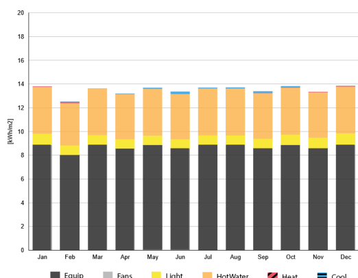
B. Intensidad del uso de energía del caso final
