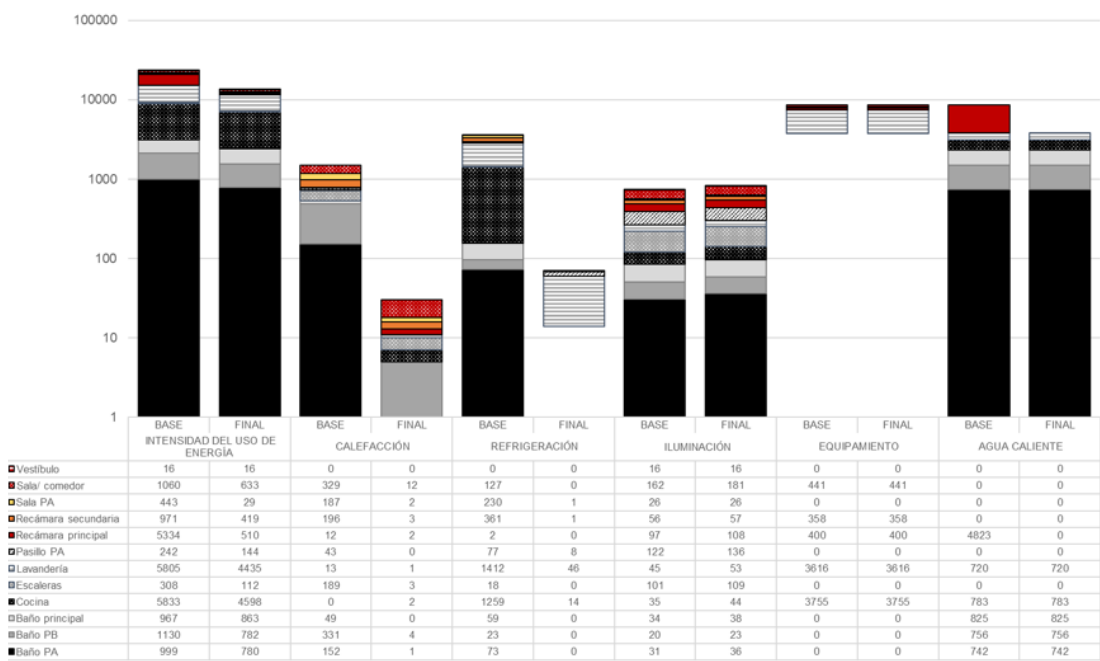
FIGURA 7. RESULTADOS POR ZONAS: CASO BASE EN COMPARACIÓN CON EL CASO FINAL.
