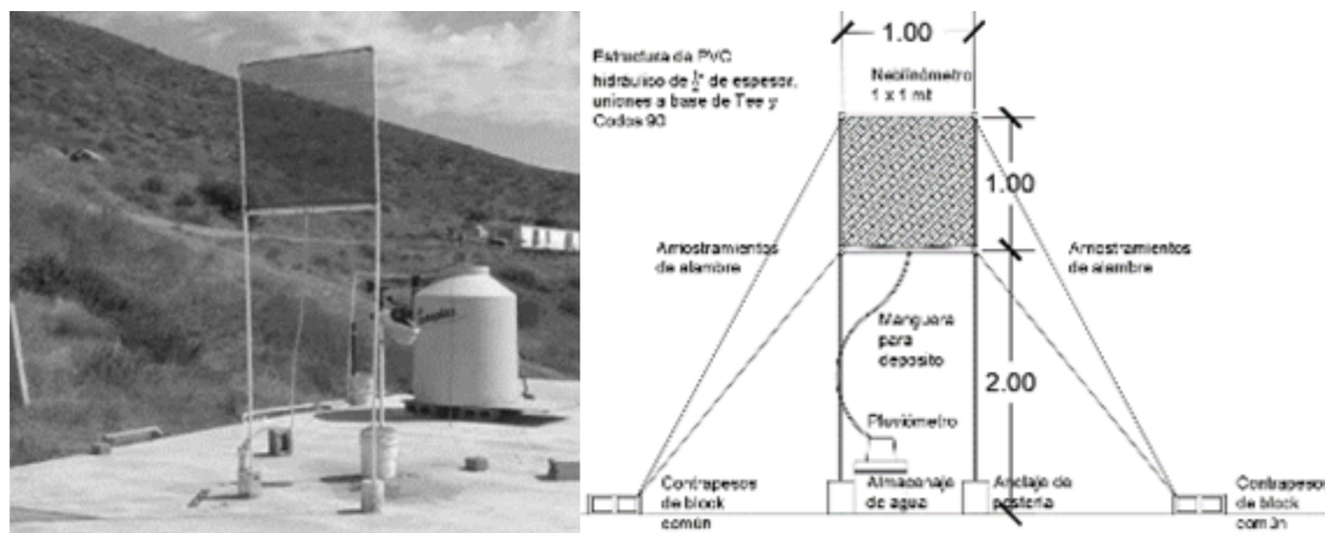
Figura 7 . Esquema de neblinómetro y puesta en sitio. Fuente: Diseño propio basado en dimensiones S. Cereceda (1994).
