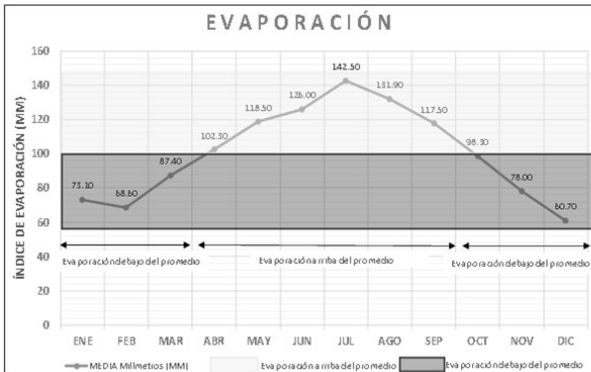
Figura 3. Índice de evaporación anual. Fuente: Datos normalizados EMA La Presa, Ensenada BC.
