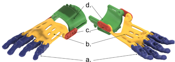
FIGURA 5. MODELO DIGITAL FINAL PRE-MANUFACTURA. A). ARTICULACIÓN DE DEDOS, B) PALMA/DORSO, C) PLACAS LATERALES Y D) BRAZALETE. FUENTE: ELABORACIÓN PROPIA GENERADA EN PROGRAMA AUTODESK FUSION 360.
