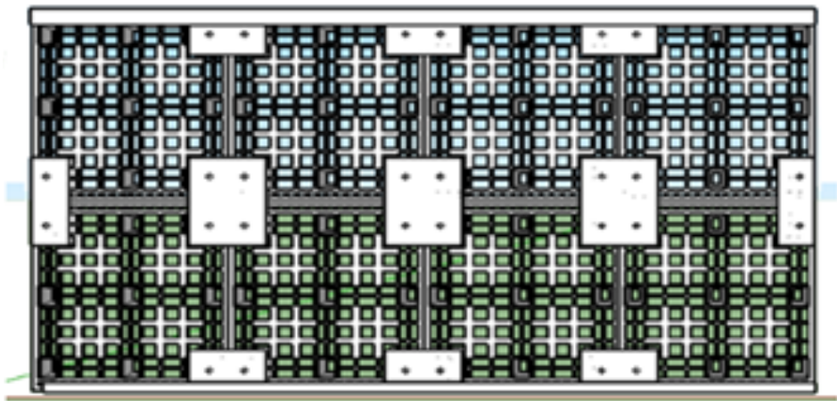
FIGURA 6. CONEXIONES DE TARIMAS. FUENTE: DIBUJO DE CASANDRA ANDREA TREJO PIMENTEL.
