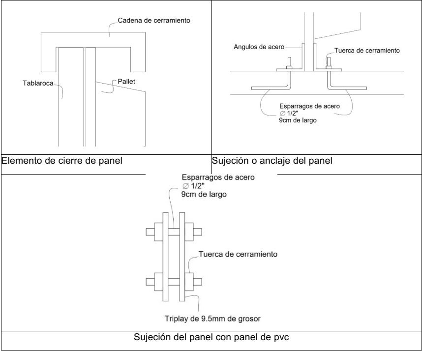
FIGURA 7. DETALLES DE CONEXIÓN Y UNIÓN ENTRE TARIMAS Y SUJECIÓN INFERIOR Y SUPERIOR DEL MÓDULO.
