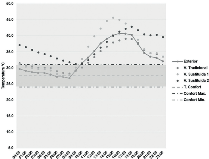
FIGURA 7. COMPORTAMIENTO TÉRMICO EN TEMPORADA 1 LA SUBIDA.
