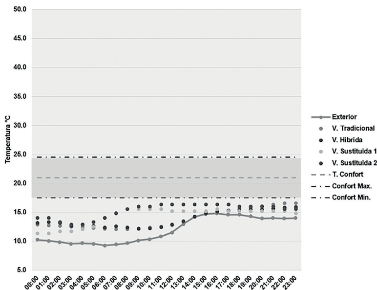
FIGURA 5. COMPORTAMIENTO TÉRMICO EN TEMPORADA 2 LA LIMA.
