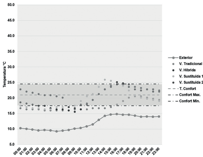
FIGURA 11. COMPORTAMIENTO TÉRMICO EN TEMPORADA 1 RANCHO NUEVO. FUENTE: DESEMPEÑO AMBIENTAL DE LA VIVIENDA RURAL, MICRORREGIÓN HUASTECA NORTE, SAN LUIS POTOSÍ. ELABORACIÓN PROPIA.
