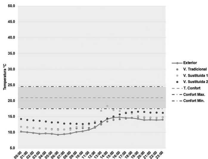
FIGURA 8. COMPORTAMIENTO TÉRMICO EN TEMPORADA 2 LA SUBIDA.
