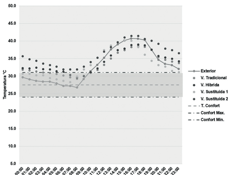
FIGURA 4. COMPORTAMIENTO TÉRMICO EN TEMPORADA 1 LA LIMA.
