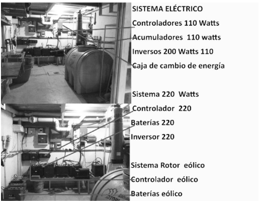
FIGURA 8. SISTEMA ELÉCTRICO.
