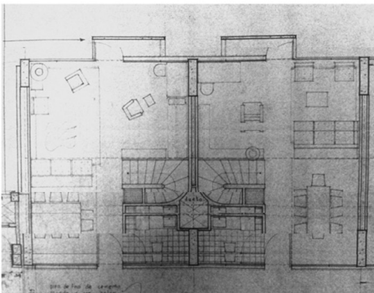
FIGURA 5. PLANTAS ARQUITECTÓNICAS DEL APARTAMENTO DÚPLEX.
