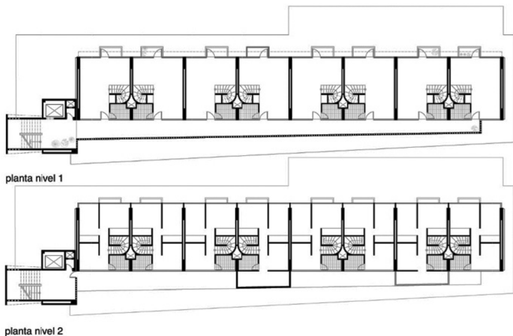
FIGURA 4. PLANTAS ARQUITECTÓNICAS DEL MULTIFAMILIAR PARA MAESTROS, 2018. SE APRECIAN LOS DOS NIVELES DEL DEPARTAMENTO TIPO DÚPLEX, ASÍ COMO LA CONSTRUCCIÓN DE TERRAZAS POR ALGUNOS VECINOS EN LAS PLANTAS SUPERIORES.
