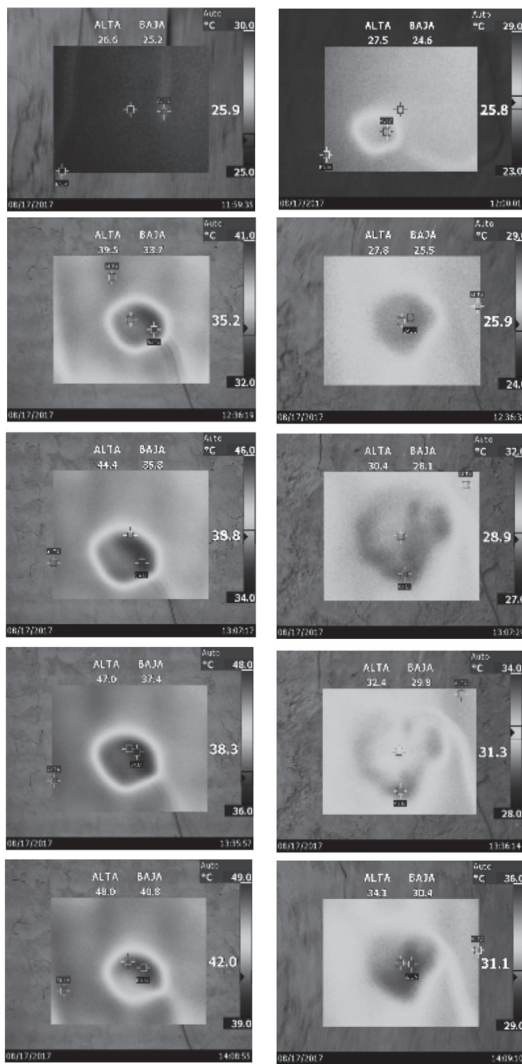
FIGURA 10. FOTOS TERMGRÁFICAS OBTENIDAS EN LA CARA ANTERIOR Y POSTERIOR DEL PANEL DE BAHAREQUE CON GRAVILLA DURANTE LA PRUEBA DE 2:30 HORAS. FUENTE: ELABORACIÓN PROPIA.
