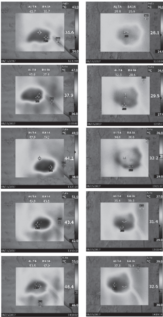
FIGURA 9. FOTOS TERMGRÁFICAS OBTENIDAS EN LA CARA ANTERIOR Y POSTERIOR DEL PANEL DE BAHAREQUE CON FIBRAS DURANTE LA PRUEBA DE 2:30 HORAS.
