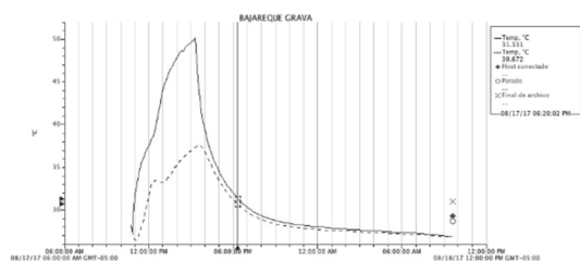
GRÁFICA 3. TEMPERATURAS OBTENIDAS EN LA CARA EXTERIOR E INTERIOR DEL PANEL DE BAHAREQUE CON GRAVILLA DURANTE LA PRUEBA DE 5 HORAS.
