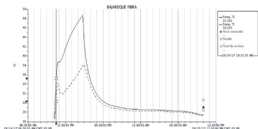
GRÁFICA 2. TEMPERATURAS OBTENIDAS EN LA CARA EXTERIOR E INTERIOR DEL PANEL DE BAHAREQUE CON FIBRA DURANTE LA PRUEBA DE 5 HORAS.
