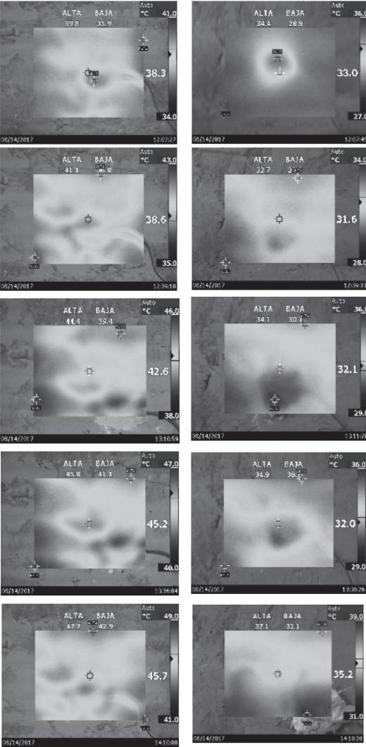
FIGURA 8. FOTOS TERMGRÁFICAS OBTENIDAS EN LA CARA ANTERIOR Y POSTERIOR DEL PANEL DE BAHAREQUE CONTROL DURANTE LA PRUEBA DE 2:30 HORAS.
