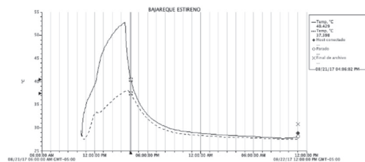
GRÁFICA 4. TEMPERATURAS OBTENIDAS EN LA CARA EXTERIOR E INTERIOR DEL PANEL DE BAHAREQUE CON POLIESTIRENO DURANTE LA PRUEBA DE 5 HORAS.
