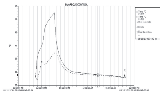
GRÁFICA 1. TEMPERATURAS OBTENIDAS EN LA CARA EXTERIOR E INTERIOR DEL PANEL DE BAHAREQUE DE CONTROL DURANTE LA PRUEBA DE 5 HORAS.
