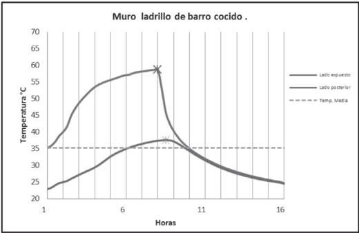
GRÁFICA 5. TEMPERATURAS OBTENIDAS EN LA CARA EXTERIOR E INTERIOR, MURO DE LADRILLO DE BARRO RECOCIDO.
