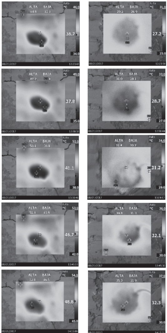
FIGURA 11. FOTOS TERMGRÁFICAS OBTENIDAS EN LA CARA ANTERIOR Y POSTERIOR DEL PANEL DE BAHAREQUE CON POLIESTIRENO DURANTE LA PRUEBA DE 2:30 HORAS. FUENTE: ELABORACIÓN PROPIA.
