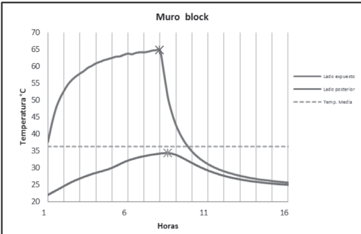
GRÁFICA 6. TEMPERATURAS OBTENIDAS EN LA CARA EXTERIOR E INTERIOR, MURO DE BLOQUES DE CONCRETO.
