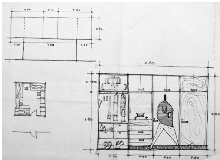
FIGURA 3. CROQUIS DE CÉLULA DE HABITACIÓN MÁS DESARROLLADA, CA. 1951. SE OBSERVA QUE LA CÉLULA SE PENSÓ PARA TRES ESTUDIANTES Y QUE EL MOBILIARIO JUGÓ UNA PARTE IMPORTANTE EN EL DISEÑO DEL ESPACIO.
