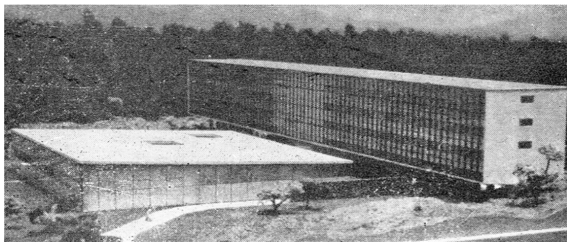
FIGURA 6. ARTÍCULO “HABITACIONES TIPO PARA ESTUDIANTES” PUBLICADO EN ARQUITECTURA MÉXICO 39. SE OBSERVA QUE LA UNIDAD TIPO SE COMPONE DE DOS ELEMENTOS PRINCIPALES, EL CUERPO DE VIVIENDA DE CINCO NIVELES Y EL APÉNDICE DE SERVICIOS DE UN NIVEL CON MEZZANINE.
