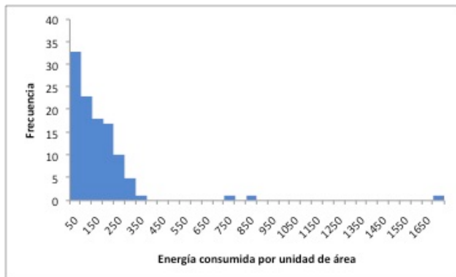
Figura 1. Histograma de la energía consumida por unidad de área para el clima cálido seco extremoso con acondicionador de aire.
